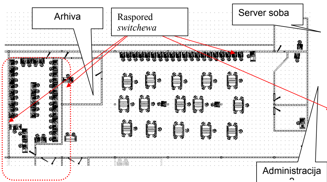
Slika broj 14 – Tlocrt prostorija u GCB-u
